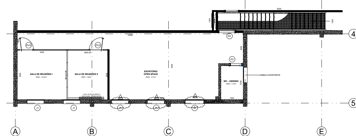
PLANTA BAIXA - 1º PAVIMENTO - ESCRITÓRIO
